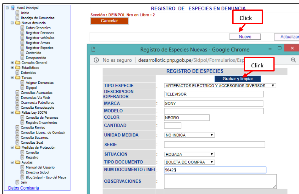
Ilustración 42: Registrar especies
