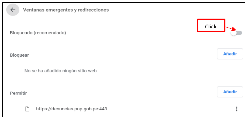
Ilustración 117: Bloqueado
