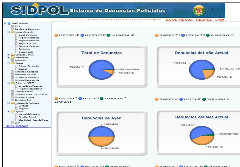
Ilustración 6: Menú principal
