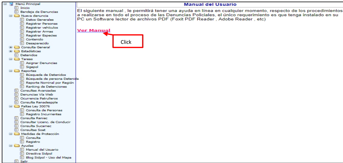
Ilustración 130: Ayudas
