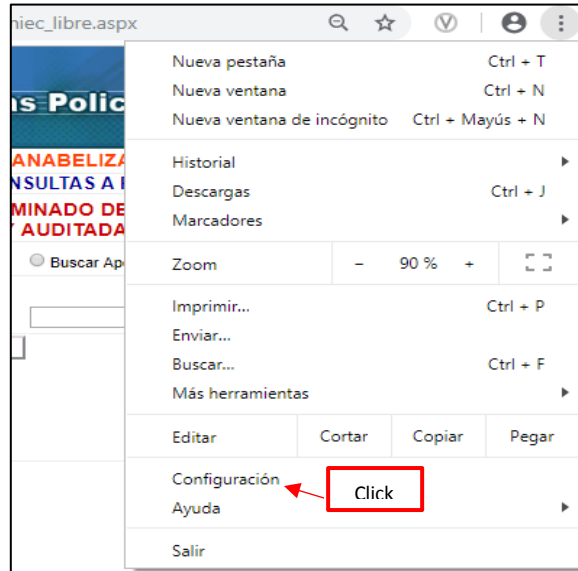
Ilustración 113: Configuración
