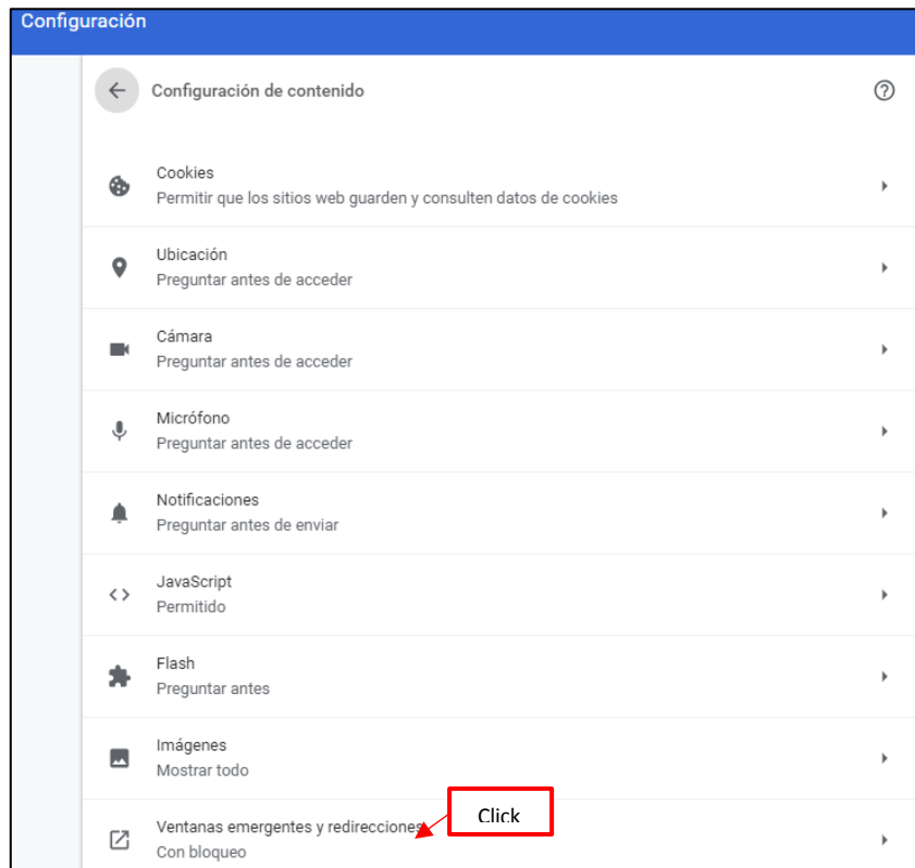
Ilustración 116: Ventanas emergentes
