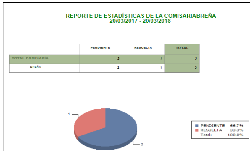
Ilustración 81: Reporte estadístico
