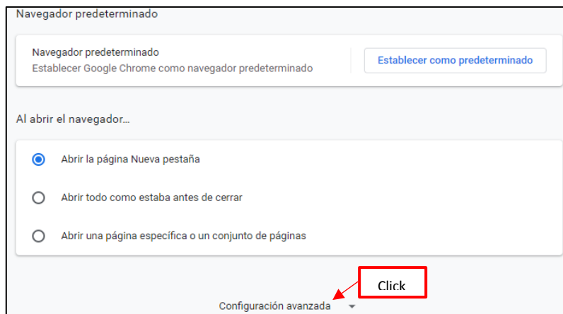
Ilustración 114: Configuración Avanzada
